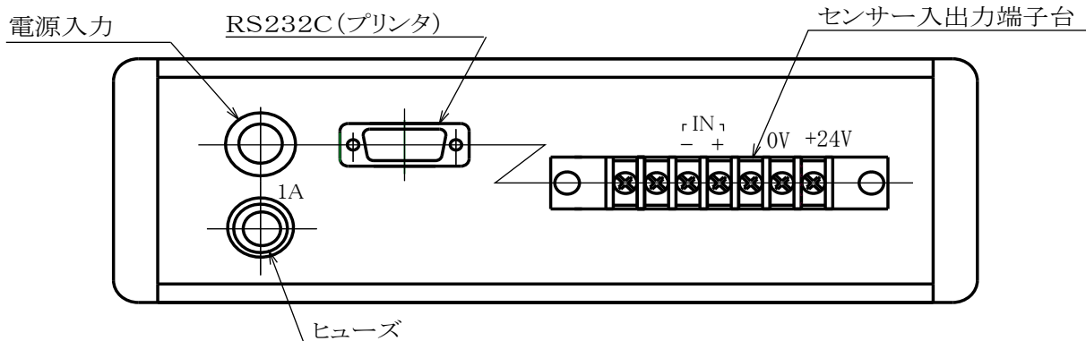
拡大背面図
