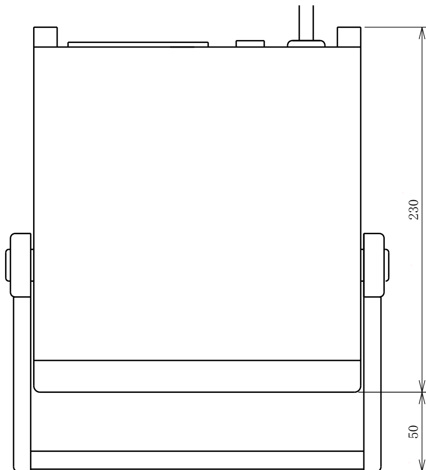
拡大背面図
