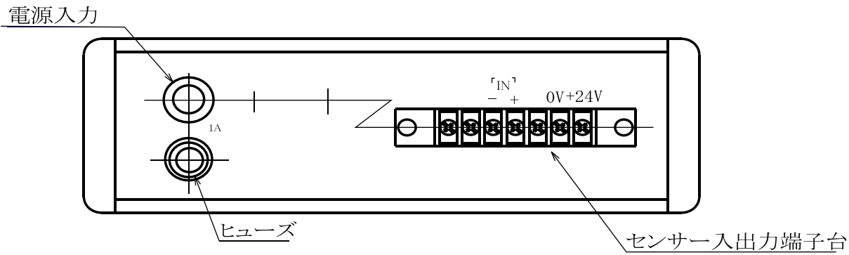
拡大背面図
