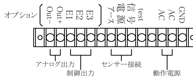
背面端子台仕様
