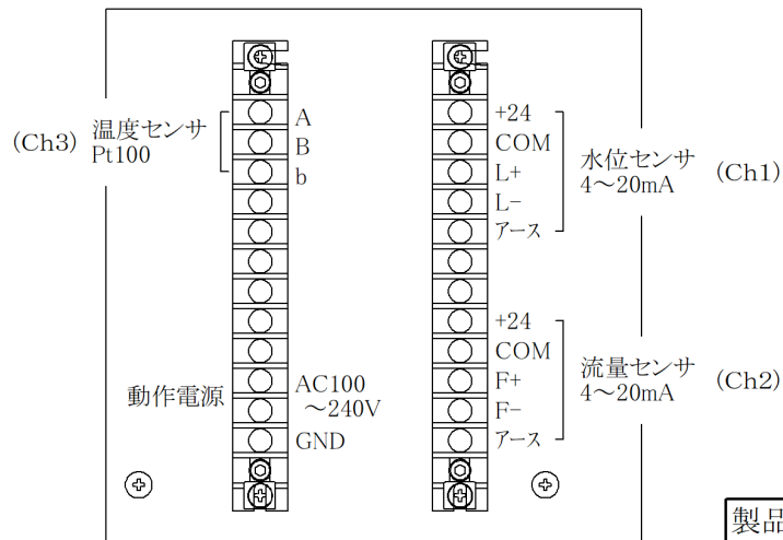
背面図
